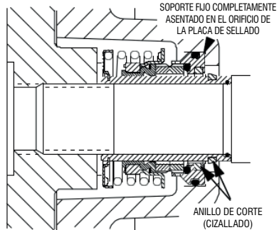
Figura 6. Sello completamente instalado
