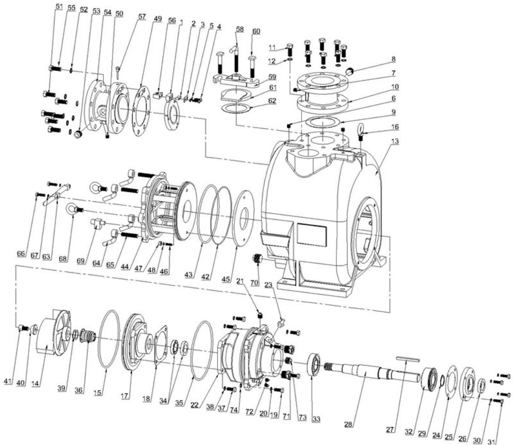
* Figura 1. Modelo de la Bomba ESPT4
