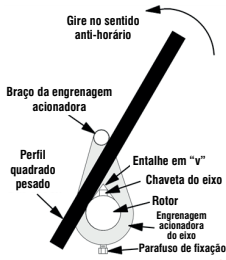
Figura 2. Afrouçamento do rotor
