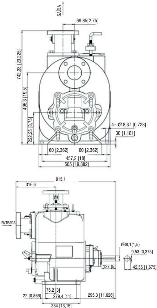
Figura 1. Bomba Modelo ESPT4
