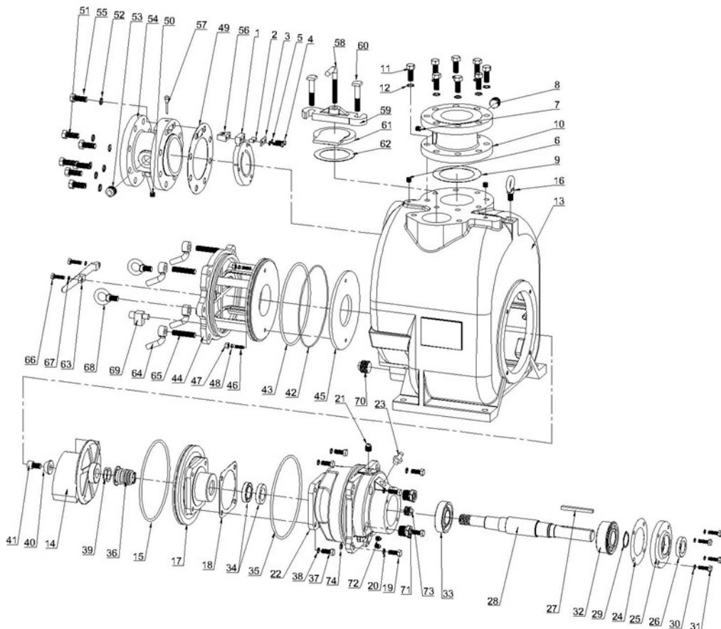
* Figura 1. Bomba Modelo ESPT4
