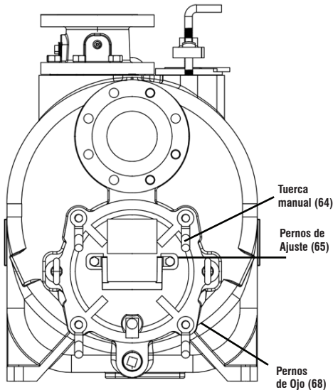
Figura 7. Instalación y ajuste de la tapa trasera
