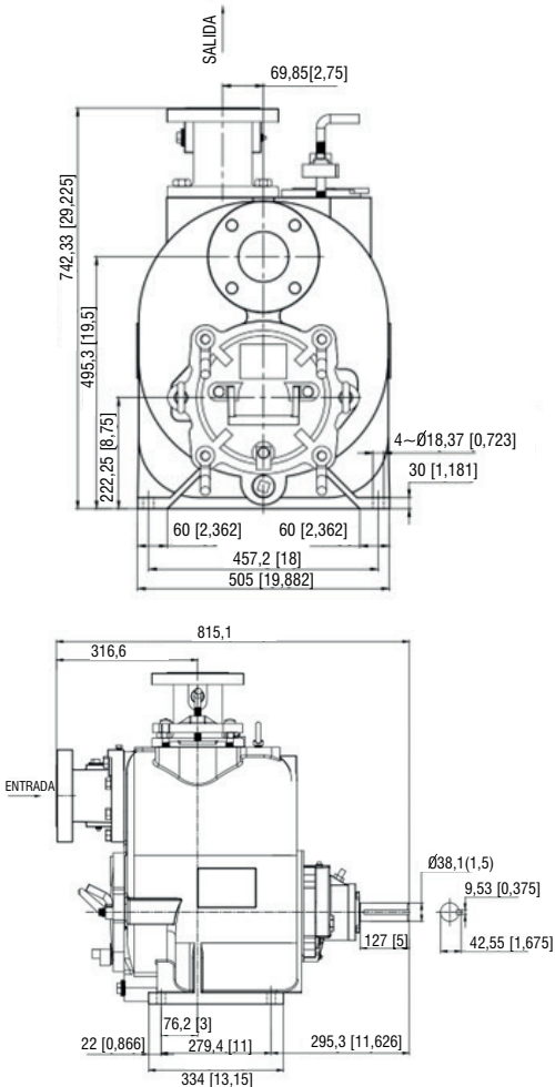
Figura 1. Modelo de la Bomba ESPT4
