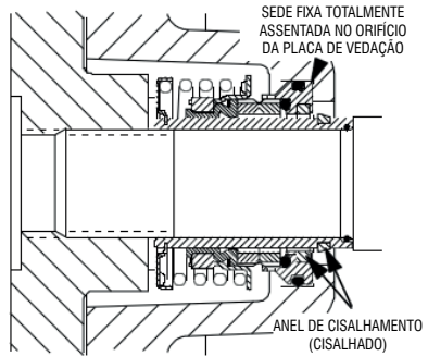
Figura 6. Selo totalmente instalado
