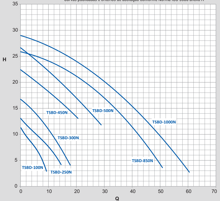
Curvas publicadas e critérios de aceitação conforme Norma ISO 9906 anexo A
