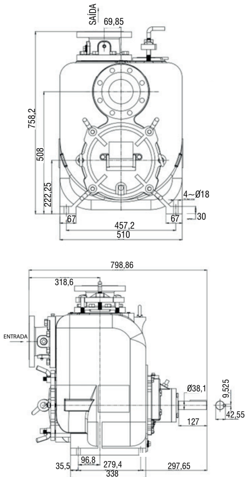
Figura 1. Bomba Modelo ESPU4
