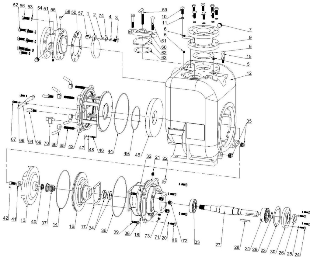
* Figura 1. Bomba Modelo ESPU4
