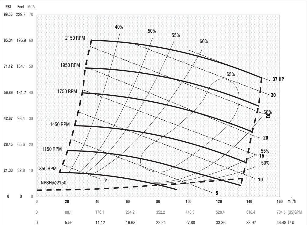
CURVA DE DESEMPENHO MODELO ESPU4
