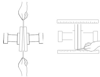
Figura 6. Alineación de Acoplamientos de Tipo No Araña
