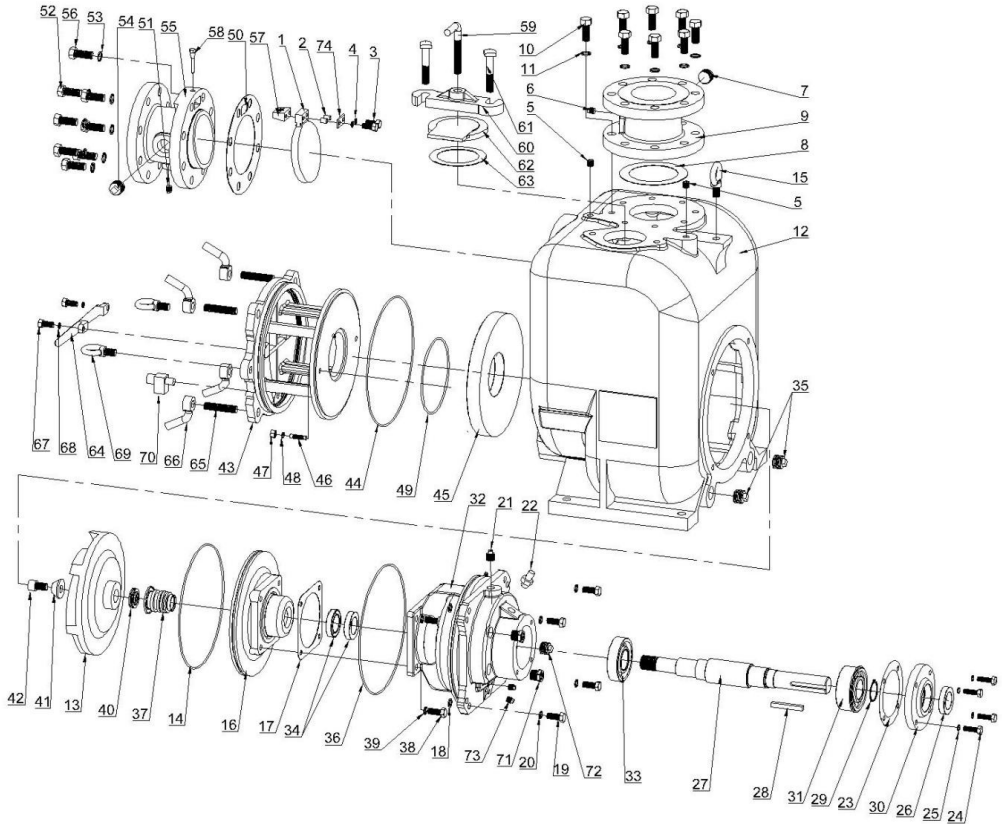
* Figura 1. Bomba Modelo ESPU4
