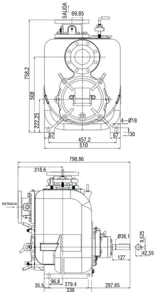
Figura 1. Modelo de la Bomba ESPU4
