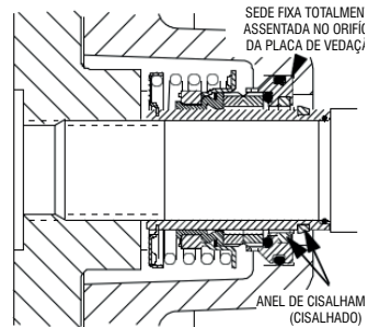
Figure 6. Selo totalmente instalado
