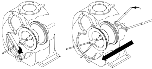
Figura 3. Extracción del conjunto giratorio
