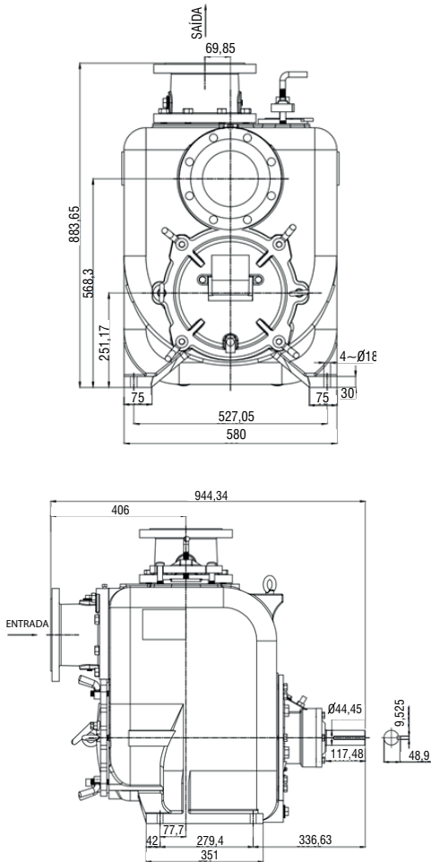
Figura 1. Bomba Modelo ESPU6
