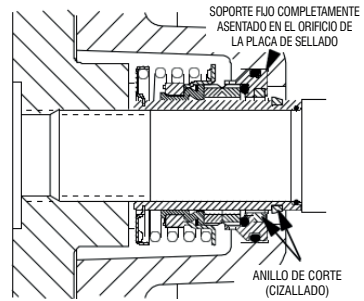
Figure 6. Selo totalmente instalado
