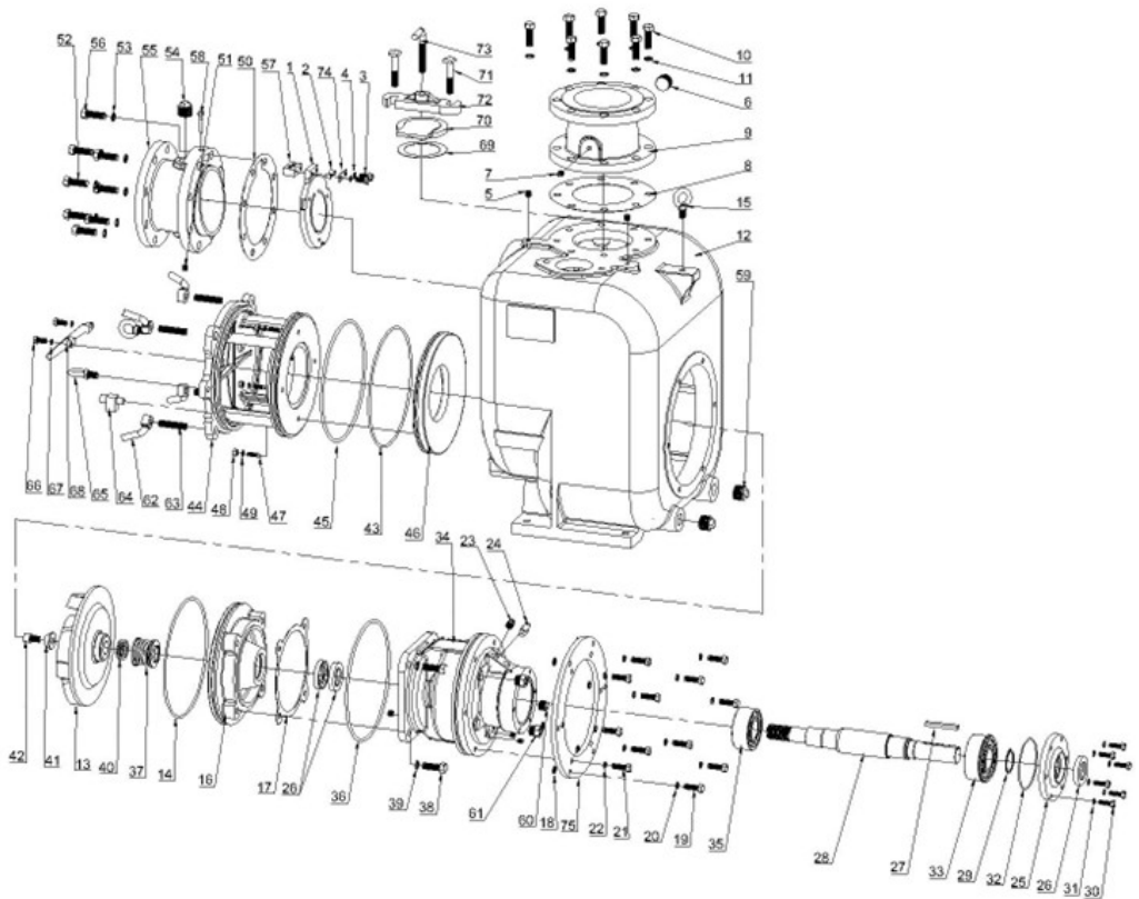
* Figura 1. Bomba Modelo ESPU6
