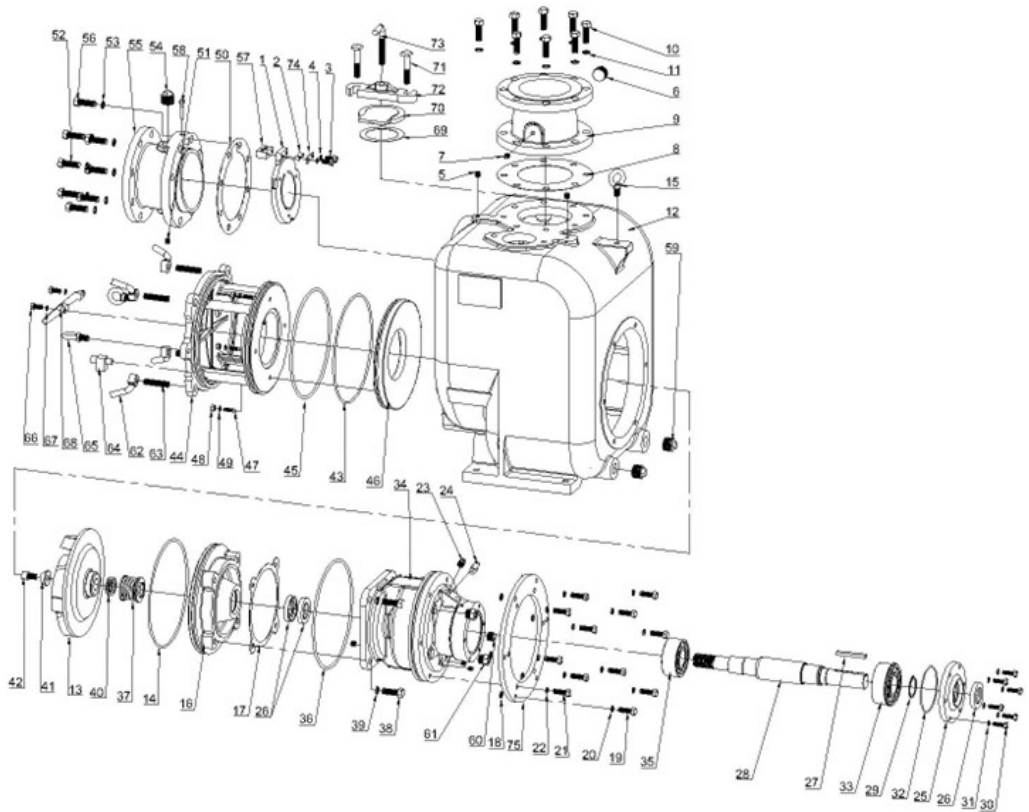
* Figura 1. Modelo de la Bomba ESPU6
