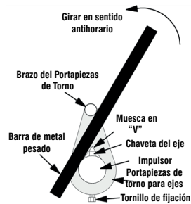
Figura 2. Aflojamiento del Impulsor
