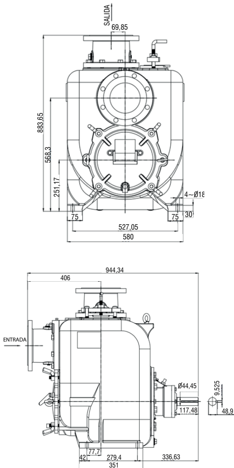
Figura 1. Modelo de la Bomba ESPU6
